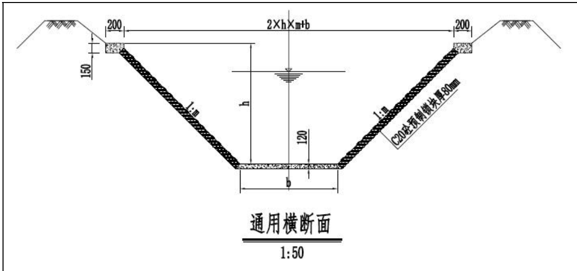
混凝土预制锁块护砌典型图
