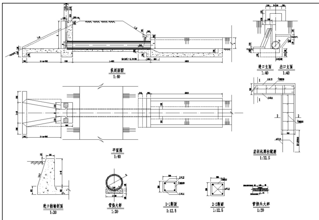
塘出水闸典型图
