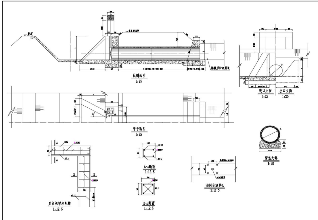
渠道进水闸典型图
