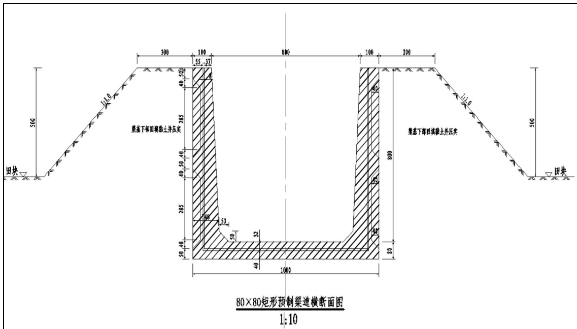
混凝土预制矩形渠典型图
