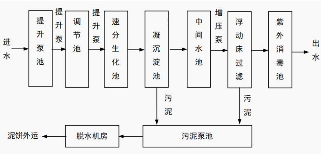
图 4-1 平桥污水处理厂处理工艺流程图
