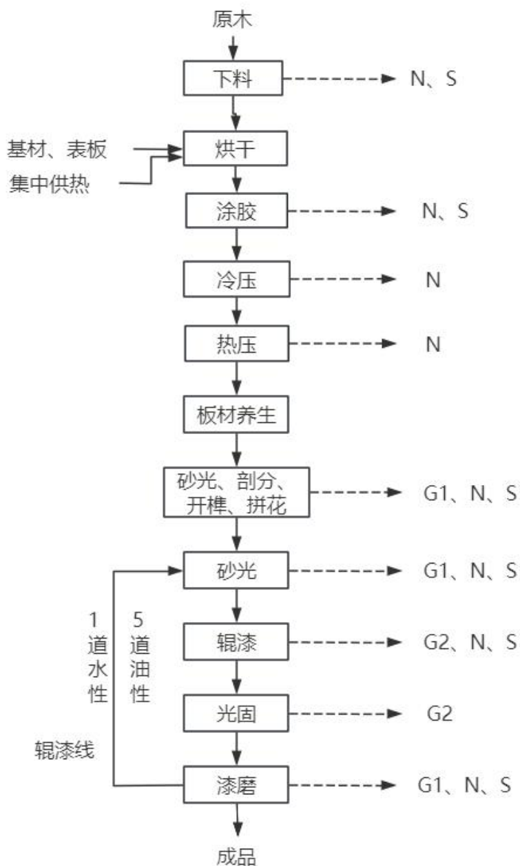
图2-2 项目木地板生产工艺及产污节点图
