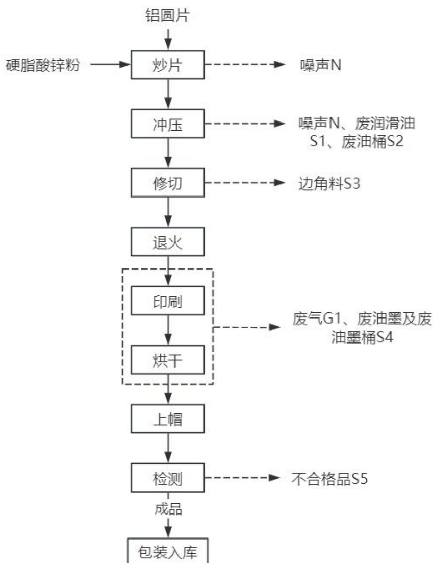
图2-2 铝管生产工艺流程及产污节点图
